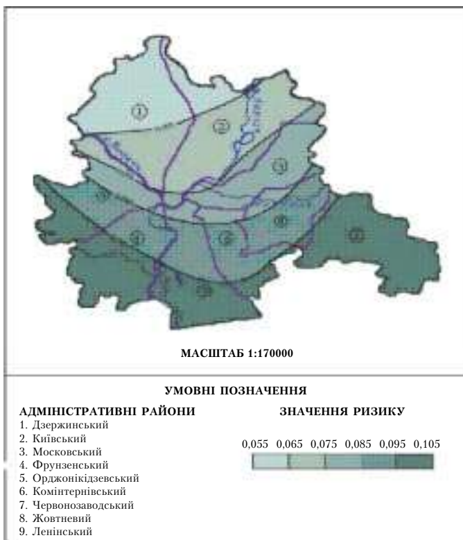
Територіальне районування сукупного індивідуального нелетального ризику за агентами діоксидазоту та формальдегіду
