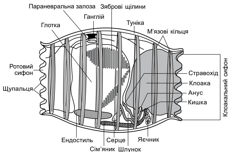
Рис. 2.8. Будова барильника
