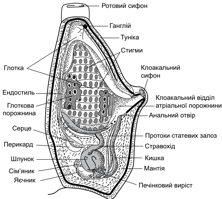
Рис. 2.2. Будова асцидії
