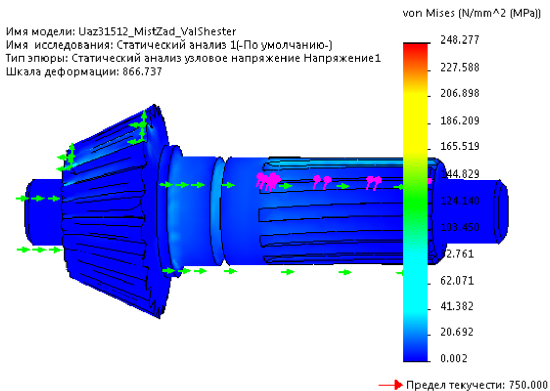
Рис. 2. Вузові напруження von Mises
