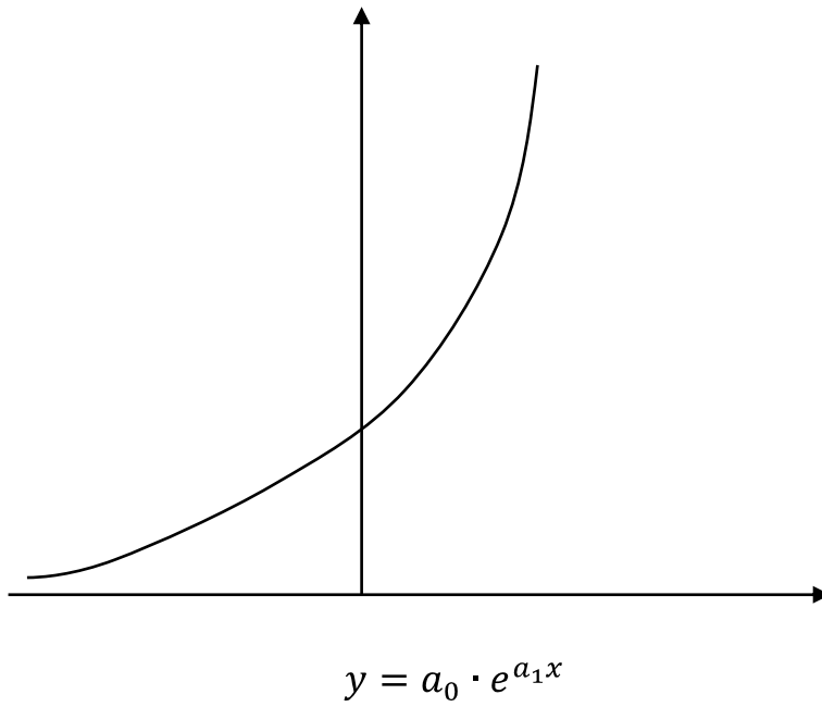
Рис. 6.2. Експоненціальний зв'язок
