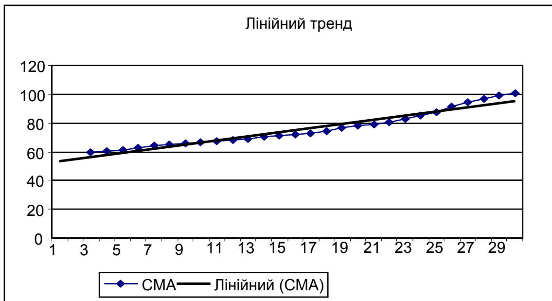
Рис. 7.7. Лінійний тренд
