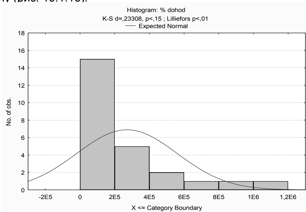
Рис. 10.1.16. Гістограма розподілу
