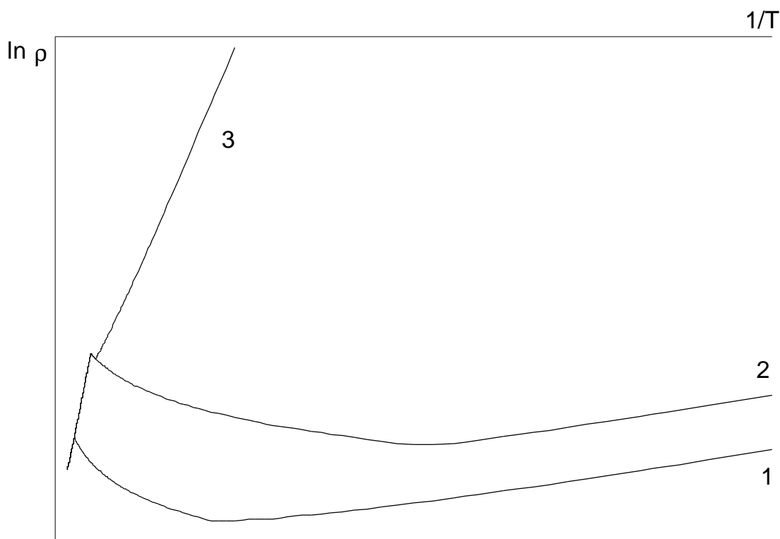
Рис. Л4.1. Схематичний вигляд температурної залежності питомого електричного опору напівпровідника, що містить легуючу донорну домішку
