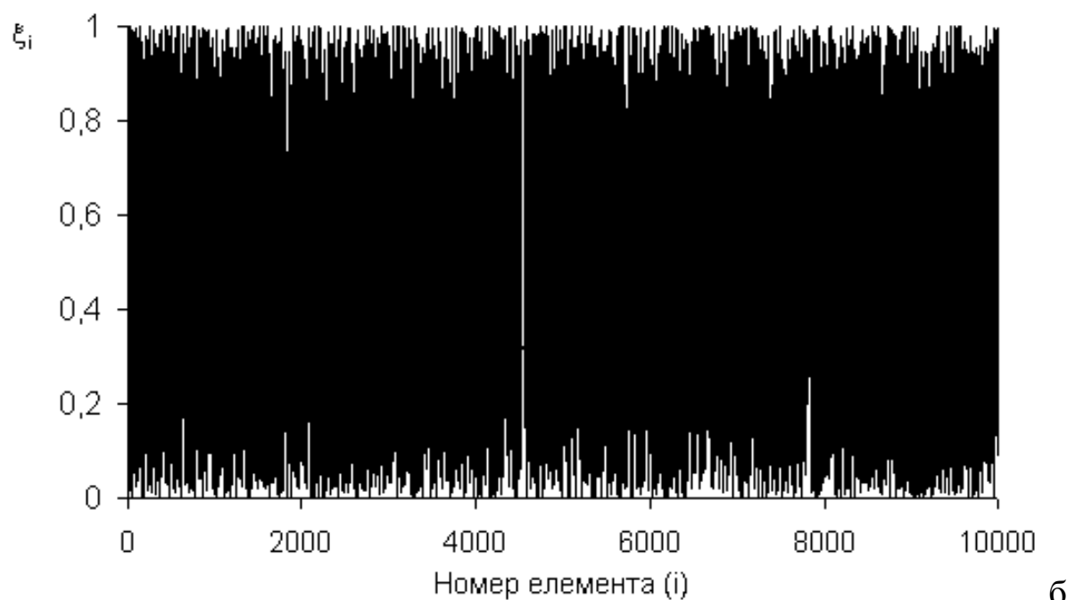
Рис. Лб.2. Діаграми послідовності значень елементів псевдовипадкової послідовності, побудованої за наведеним алгоритмом, (а) і послідовності, отриманої за допомогою пакета аналізу MS Excel, (б)
